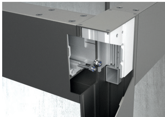
Tvåkammarbalk för dränage
